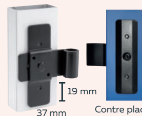
Équerre bout festonné réglable
