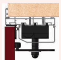
Coupe précadre et capot
