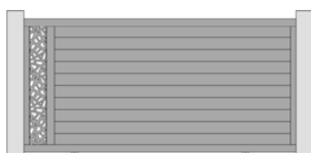
Brunelle - coulissant 1 décor vertical à gauche (vue ext.)
