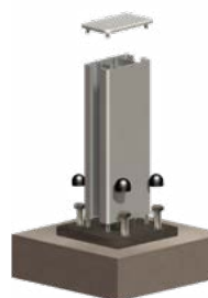
Poteau sur embase renforcée
