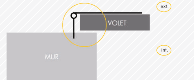
Pose en APPLIQUE Le volet se ferme par-dessus la façade en haut, à gauche, à droite
