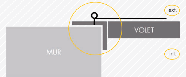
Pose en rénovation facile avec PRECADRE alu 3 côtés Le précadre recouvre les gonds coupés
