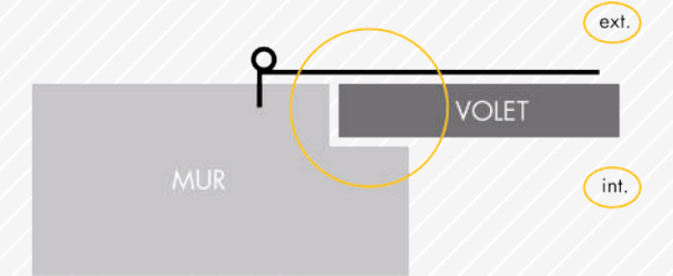
Pose en FEUILLURE Le volet se ferme dans une encoche en haut, à gauche, à droite
